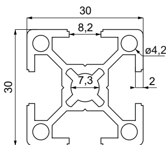
Hliníkový profil K3030 stříbrný elox
