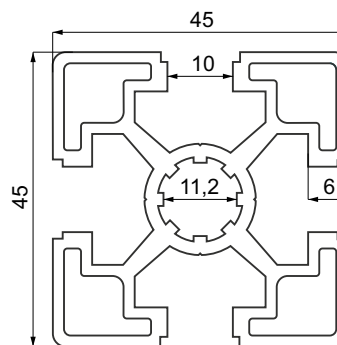
Hliníkový profil K4545 stříbrný elox
