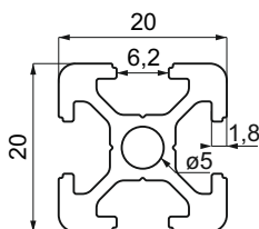
Hliníkový profil K2020 stříbrný elox
