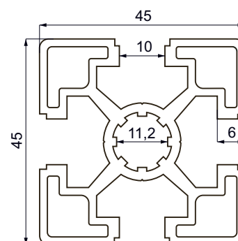
Hliníkový profil K4545 stříbrný elox
