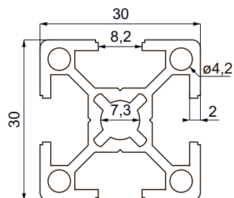
Hliníkový profil K3030 stříbrný elox Hliníkový profil K3030
