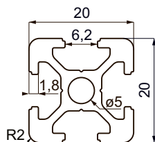
Hliníkový profil K2020 stříbrný elox
