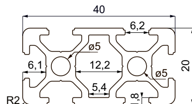
Hliníkový profil K2040 stříbrný elox
