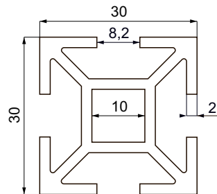
Hliníkový profil KOMBI 30 stříbrný elox Hliníkový profil KOMBI 30
