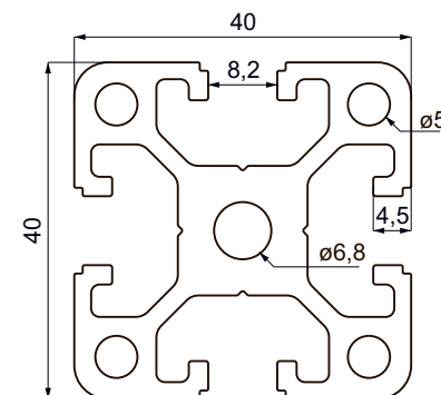
Hliníkový profil K4040 stříbrný elox
