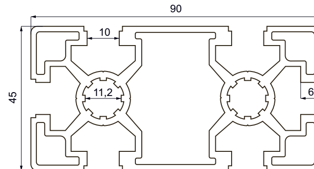
Hliníkový profil K4590 stříbrný elox
